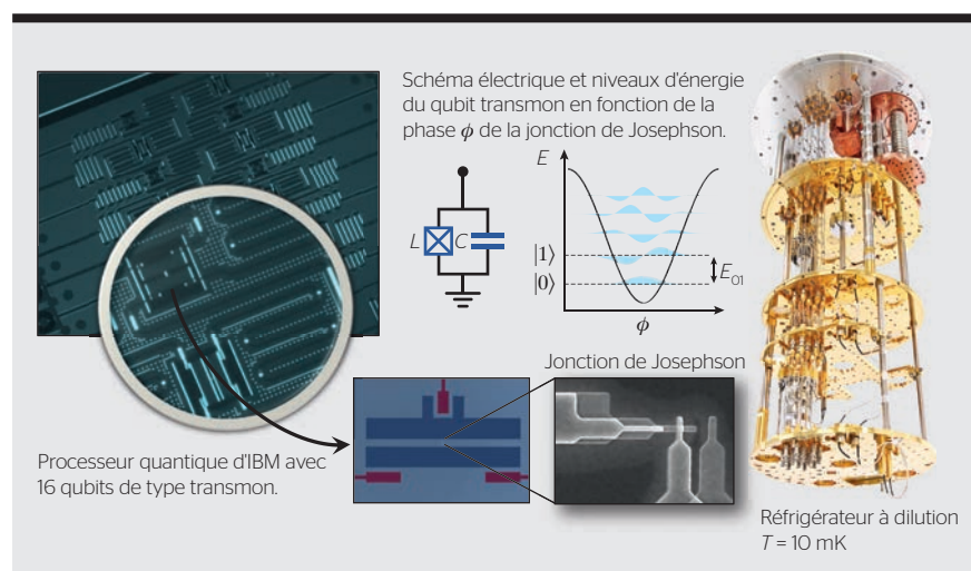
Figure 2 Plateforme de l'ordinateur quantique.
