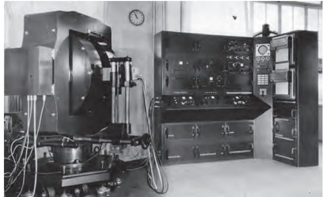
um 1963 TTC-Kernresonanz-Spektrometer KIS2, bestückt mit Elektromagnet von hoher Feldhomogenität.
