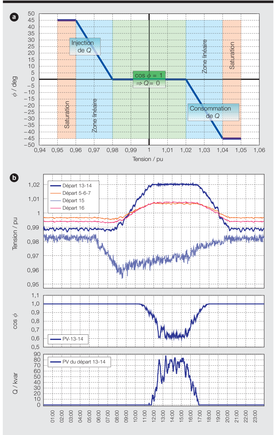
Figure 5 Loi de commande (a) et tensions dans le réseau BT choisi avec réglage par \cos \phi (b).
