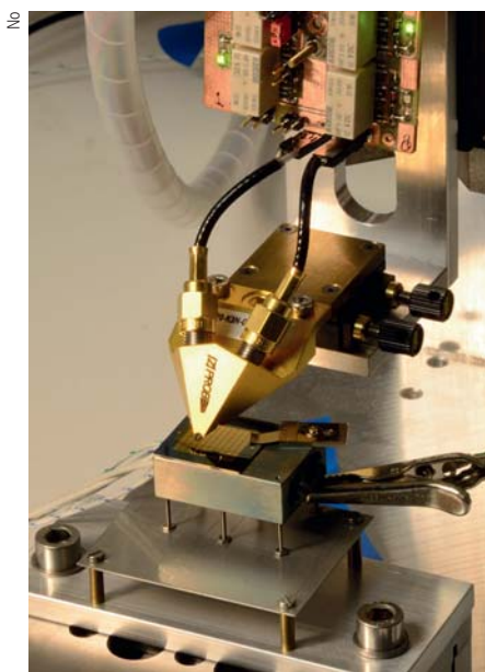
Bild 1 Probe zur Untersuchung neuer Ideen an den neusten Prototypen von Phase Change Memory Chips. Diese Chips werden im IBM-Forschungszentrum in Rüslikon hergestellt.
