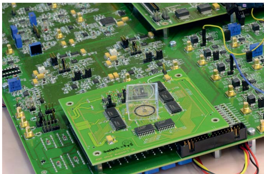
Bild 3 Plattform zum Entwickeln, Optimieren und Verifizieren von Algorithmen für das zuverlässige Schreiben und Lesen von Phase Change Memory mit Multi-Level-Möglichkeit. Der Plexiglastkasten schützt den PCM-Chip.
