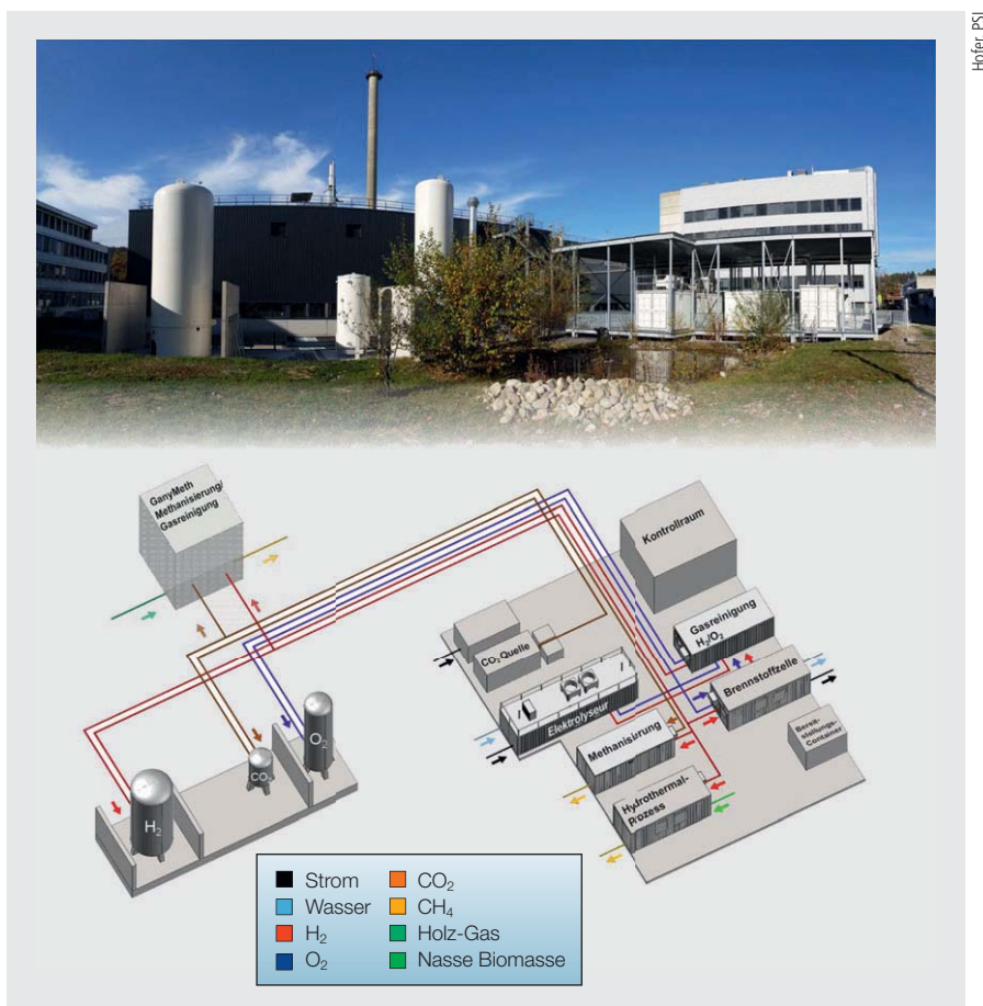
Bild 3 Energy System Integration (ESI) Plattform am Paul Scherrer Institut.
