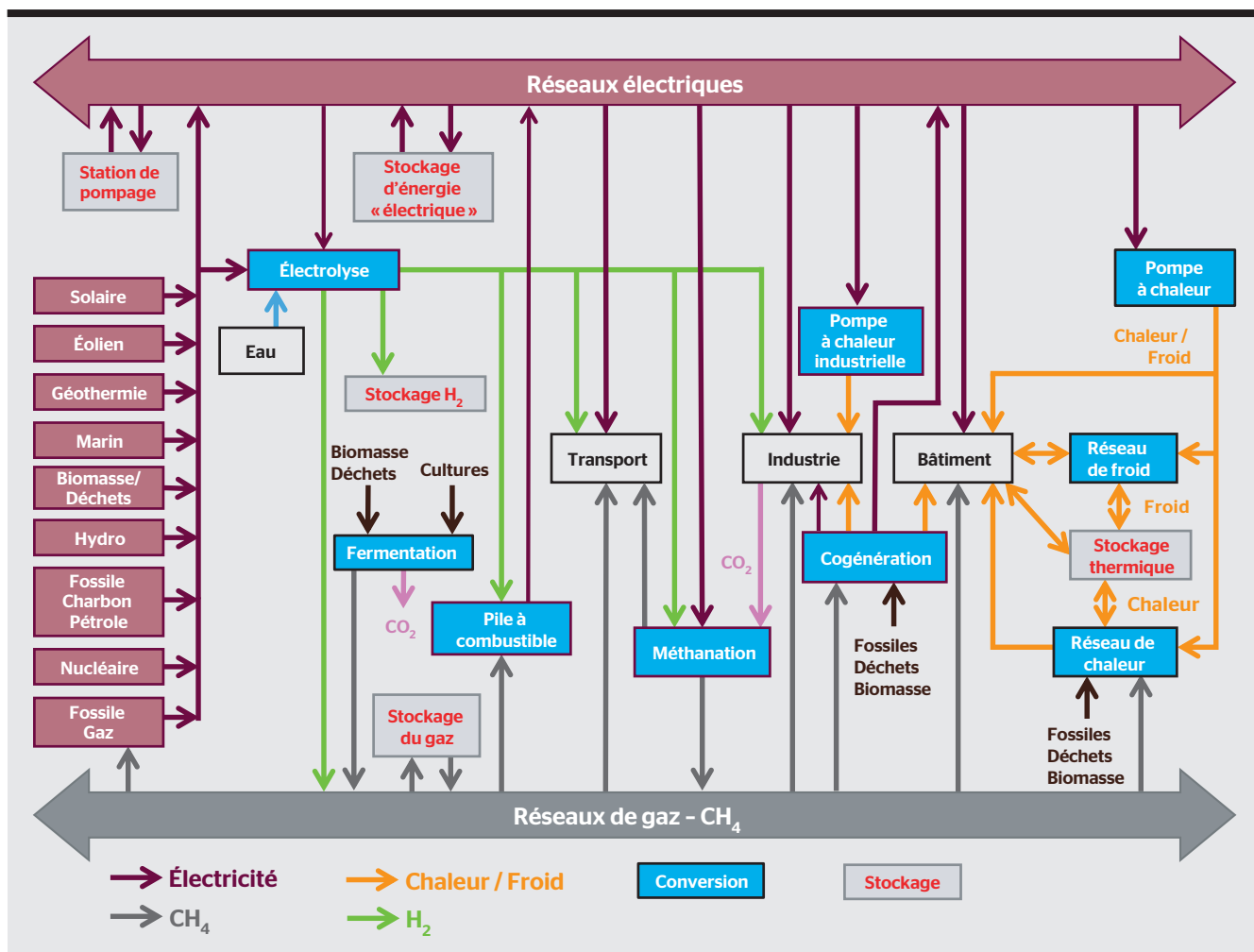
Figure 1 Systèmes multiénergies.
