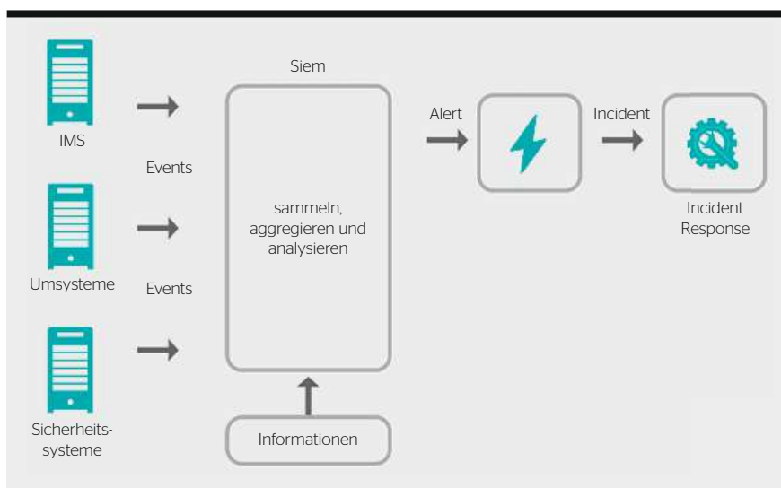
Bild 3 Events -> Alert -> Incident - was wo wie geschieht.
