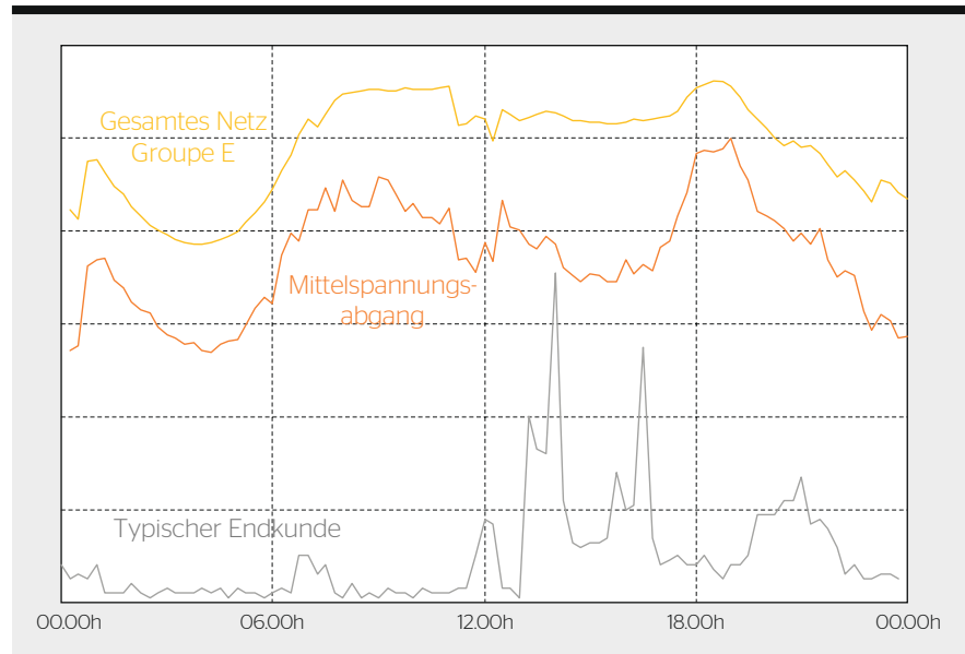
Bild 1 Typische Lastkurven im Netz von Groupe E.
