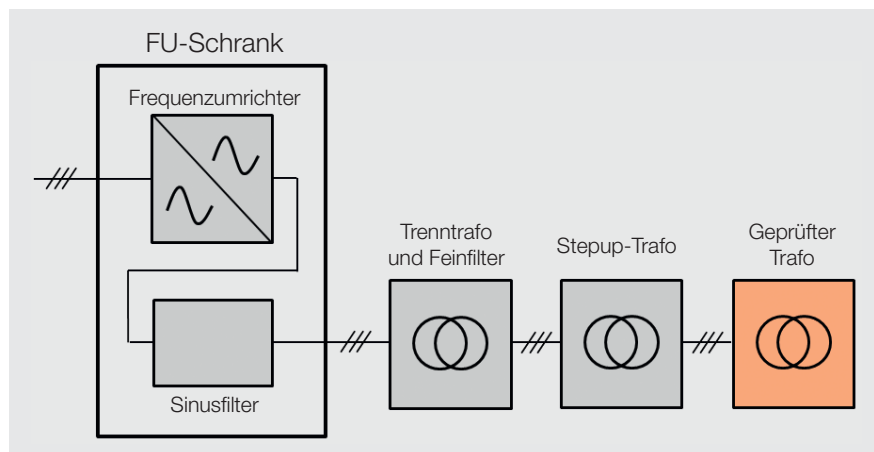
Bild 2 Prinzipschema einer Trafoprüfung mit Frequenzumrichter-Quelle.
