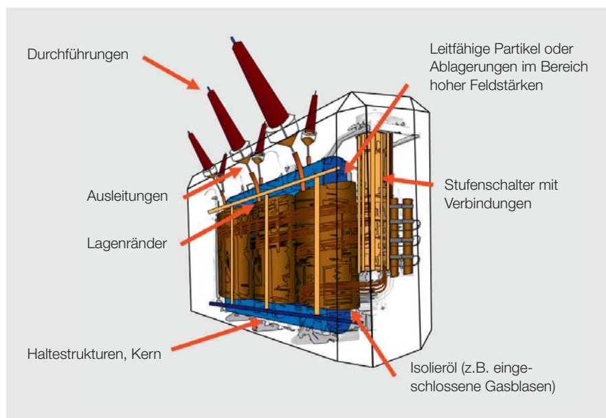
Bild 1 Häufige Teilentladungsquellen in Transformatoren.
